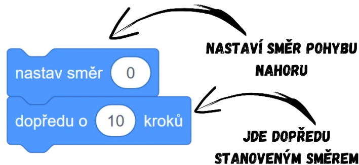
Obrázek 10 - Ukázka kódu
