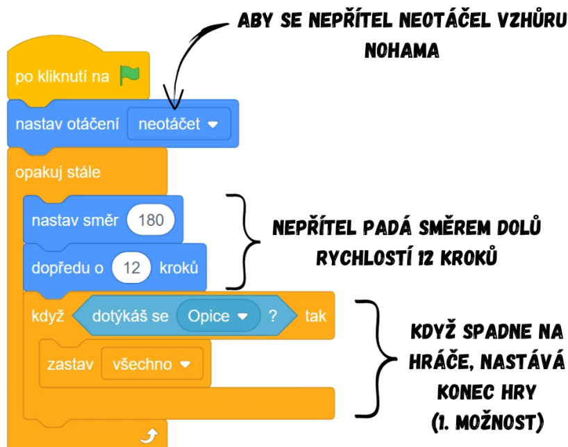
Obrázek 45 - Ukázka kódu
