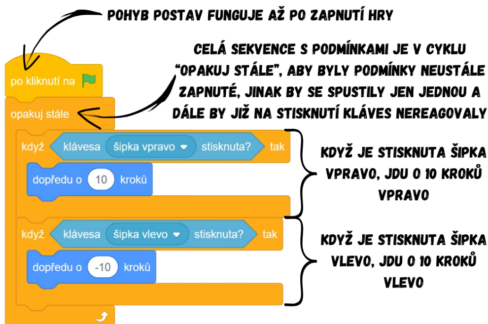
Obrázek 43 - Ukázka kódu
