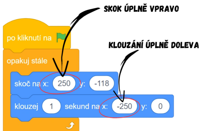
Obrázek 75 - Ukázka kódu
