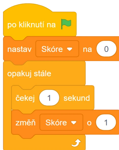
Obrázek 152 - Ukázka kódu
