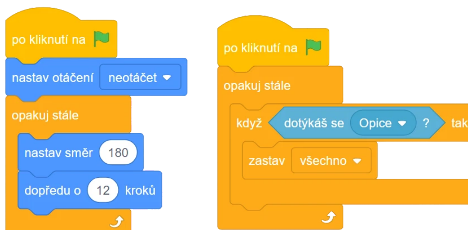
Obrázek 47 - Ukázka kódu
