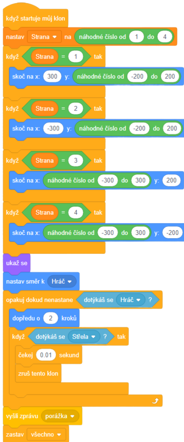
Obrázek 149 - Ukázka kódu
