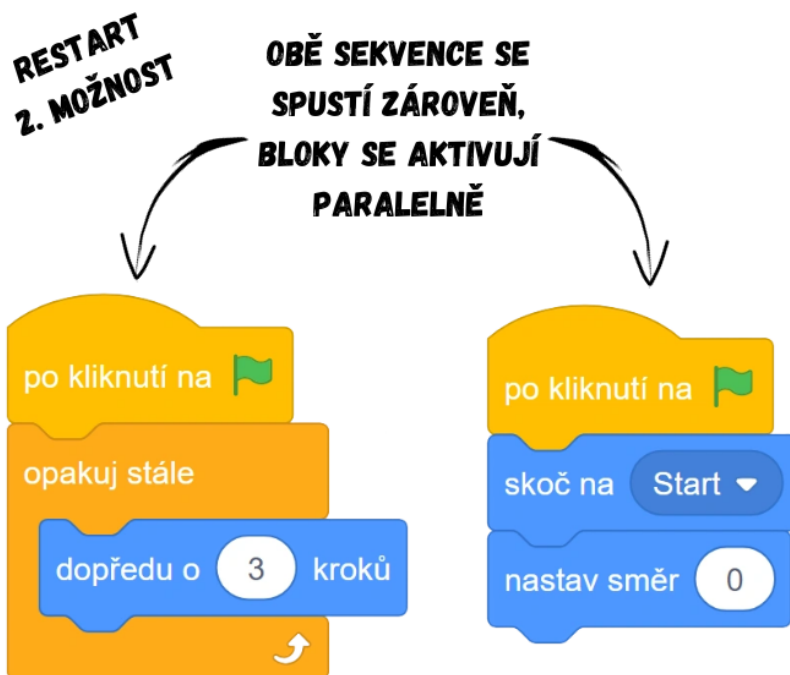
Obrázek 29 - Ukázka kódu
