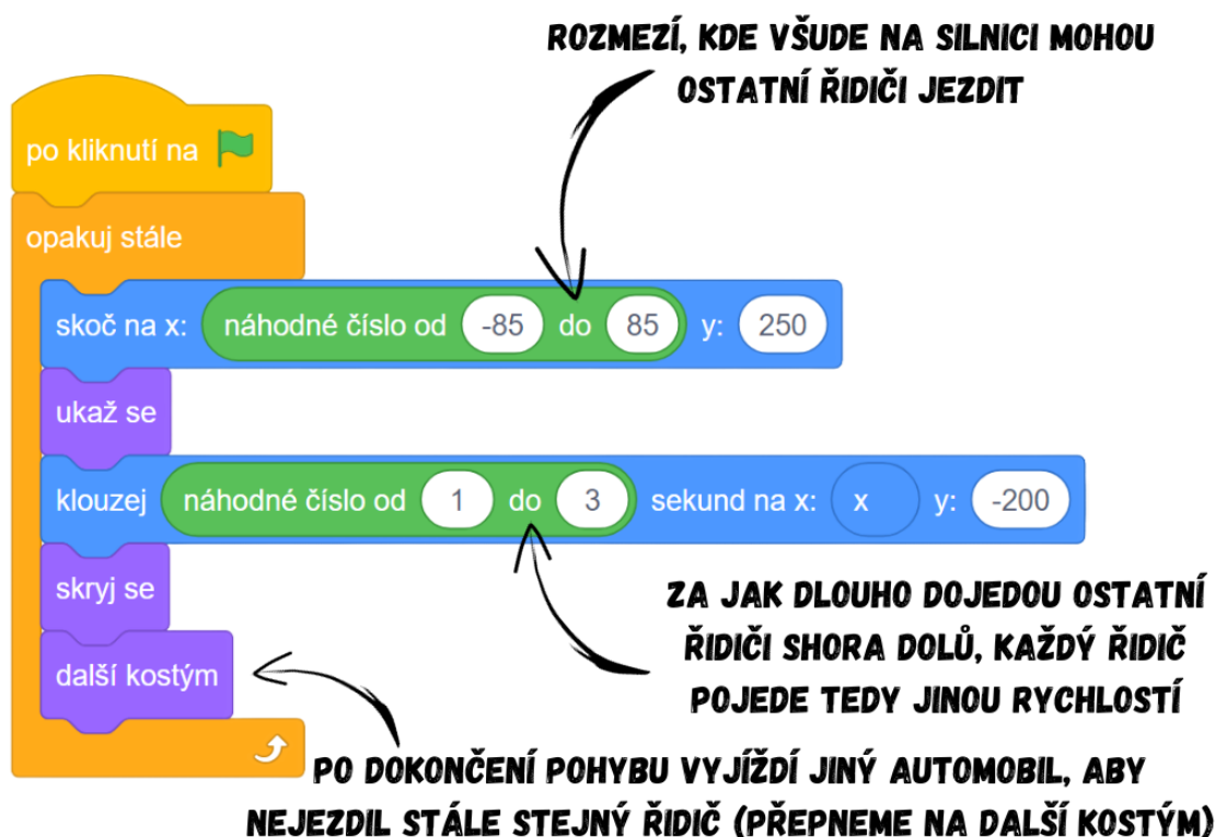
Obrázek 116 - Ukázka kódu
