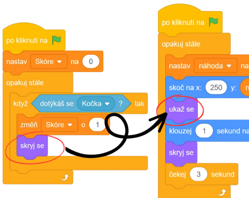
Obrázek 81 - Ukázka kódu
