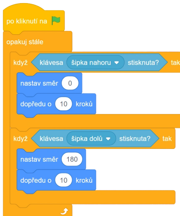
Obrázek 71 - Ukázka kódu
