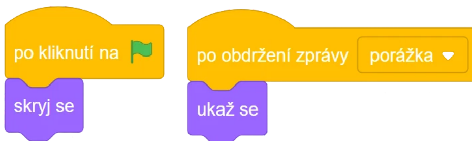
Obrázek 151 - Ukázka kódu
