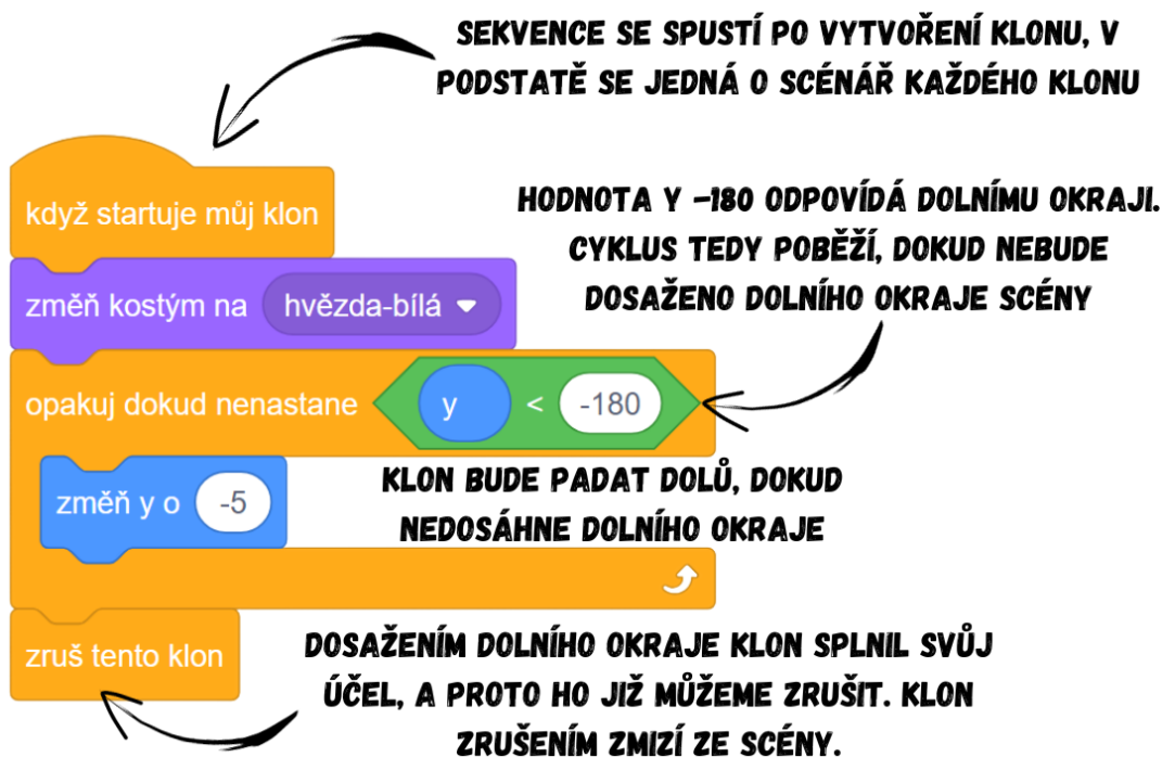
Obrázek 133 - Ukázka kódu
