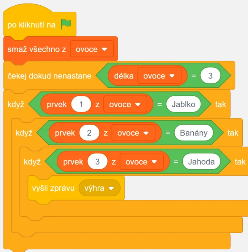
Obrázek 162 - Ukázka kódu
